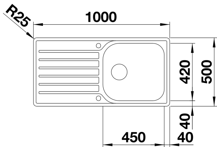
Bovenaanzicht
