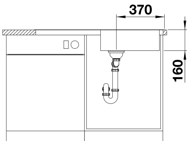
Vooraanzicht
