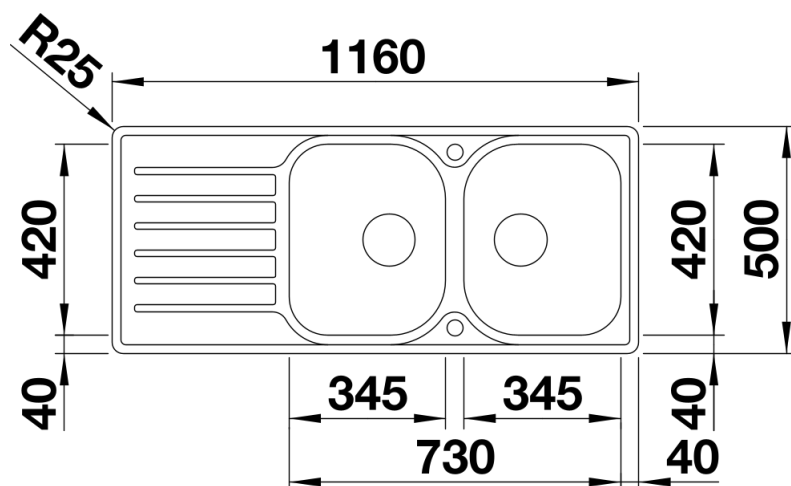
Bovenaanzicht
