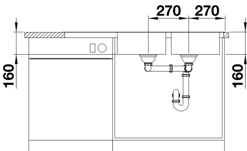
Vooraanzicht
