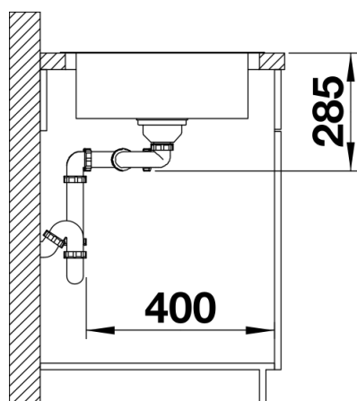
Zijaanzicht
